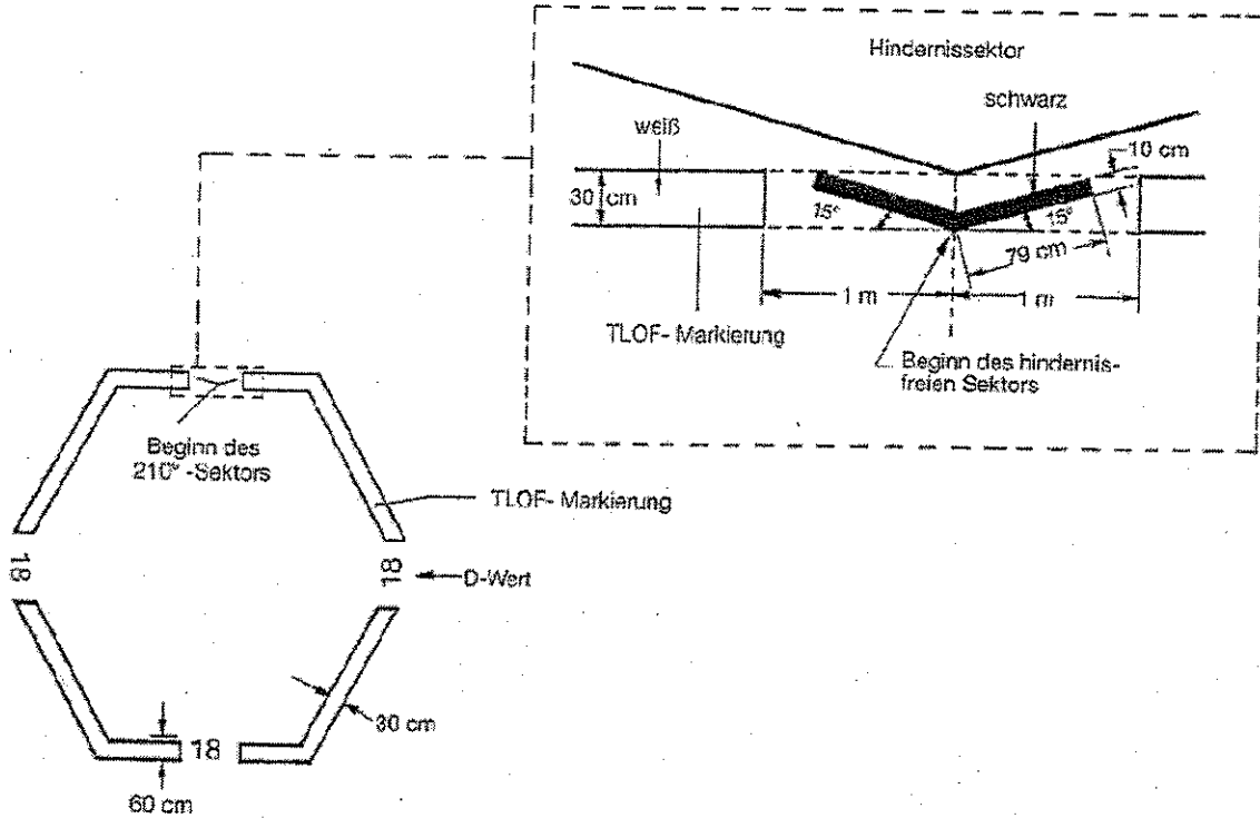
Abbildung 5-5. Markierung eines hindernisfreien Sektors eines Hubschrauberlandeplatzes
