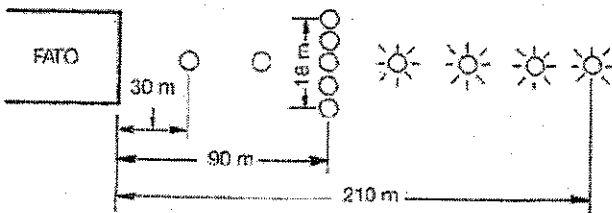
Abbildung 5-10. Anflugbefeuerung
