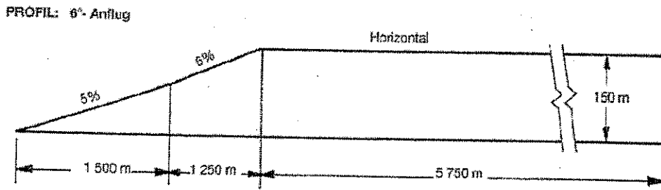
Abbildung 4-8. Anflugfläche für Präzisionsanflug-FATO
