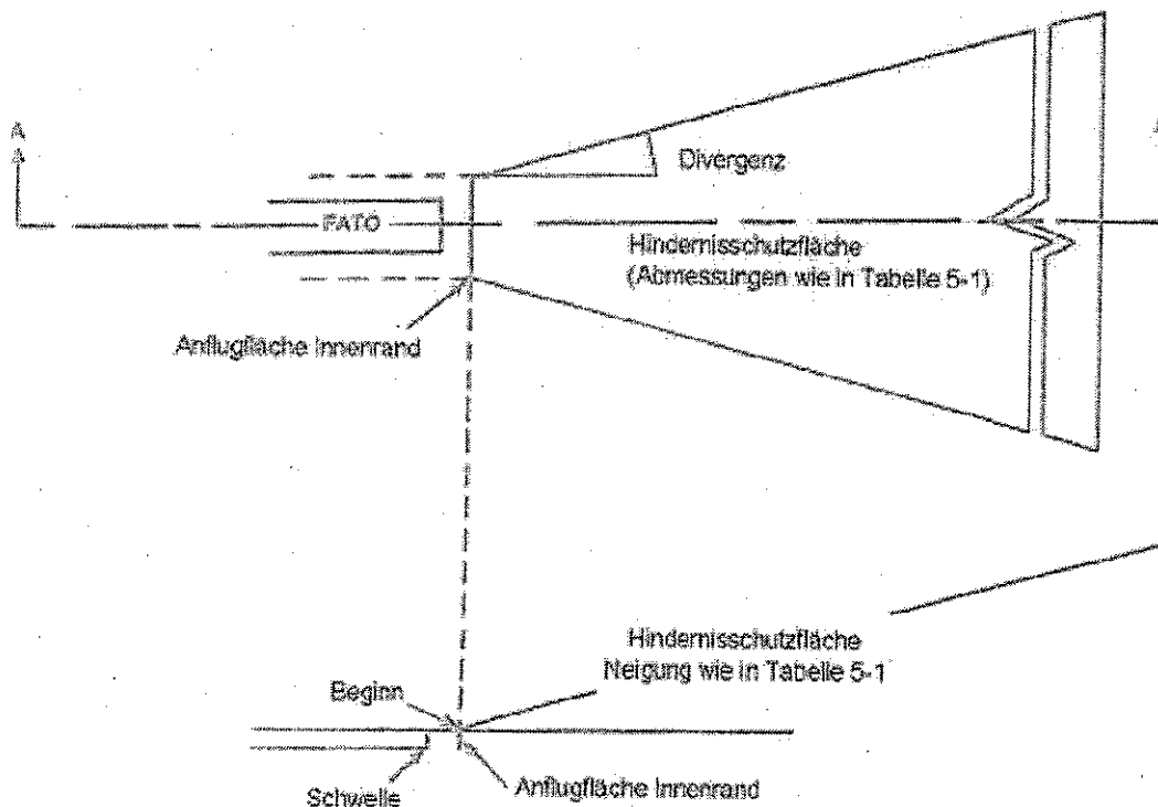
Abbildung 5-12. Hindernisschutzfläche für Gleitwinkelbefuerungen
