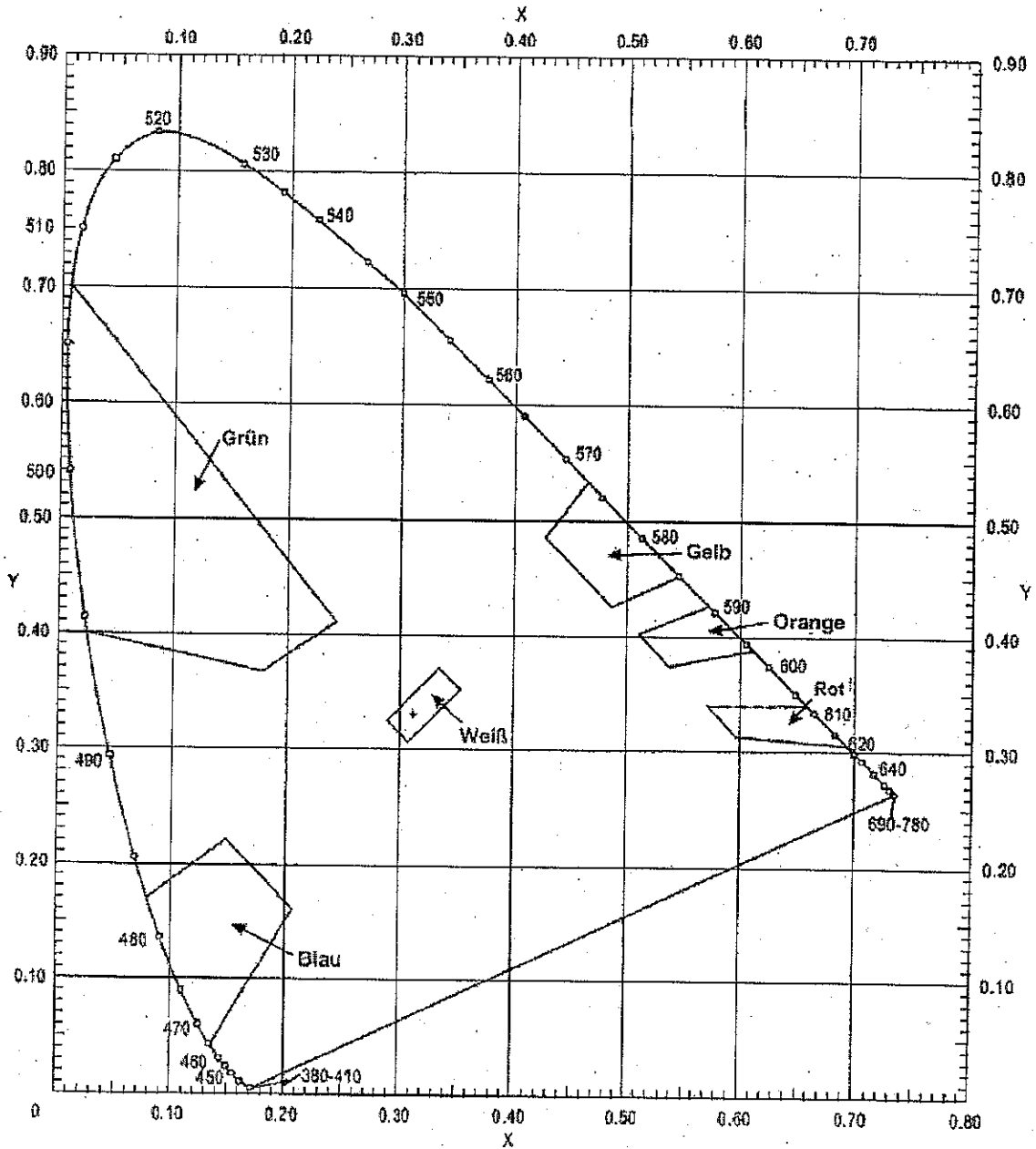
Abbildung 5-14. Farbdigramm und Leuchtdichtefaktoren für Luminiszenzplatten
