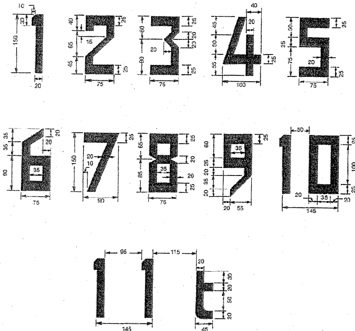
Abbildung 5-2a. Form und Größe der Zahlen und Buchstaben der Höchstmassenmarkierung
