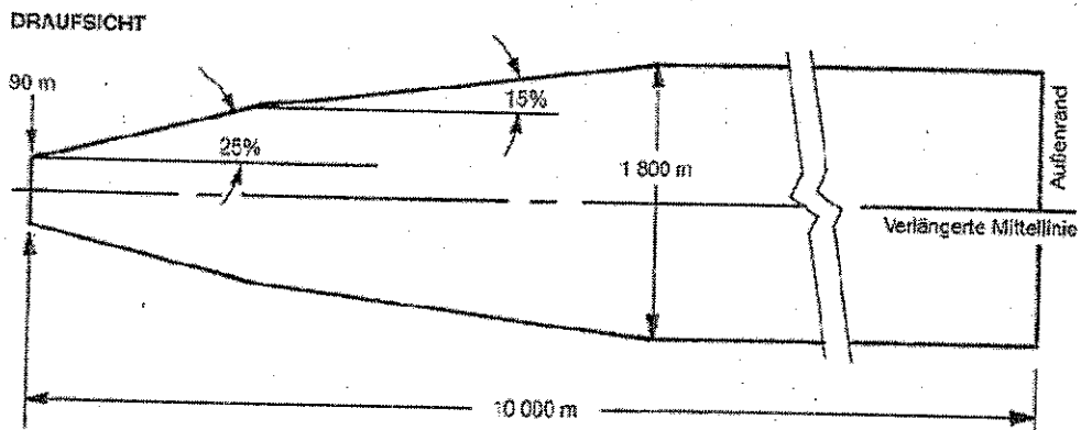
Abbildung 4-7. Abflugfläche für Instrumenten-FATO
