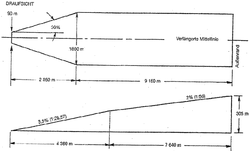
Abbildung 4-7. Abflugfläche für Instrumenten-FATO
