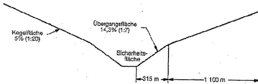
Nichtpräzisionsanflug (Endprofile)
