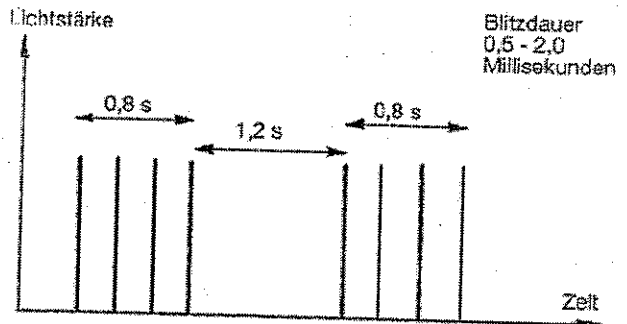
Abbildung 5-8. Blitzeigenschaften des Hubschrauberflugplatz-Leuchtfeuers
