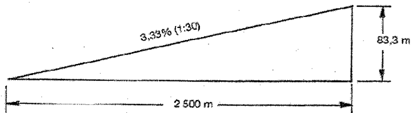
Abbildung 4-9. Anflugfläche für Nichtpräzisionsanflug-FATO
