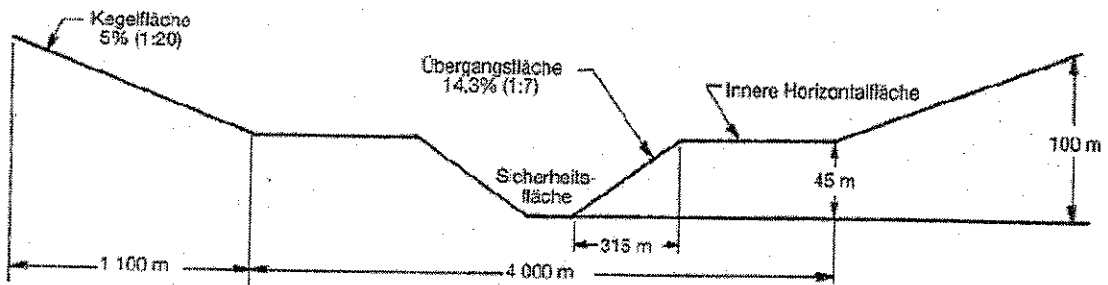
Nichtpräzisionsanflug (Endprofile)
