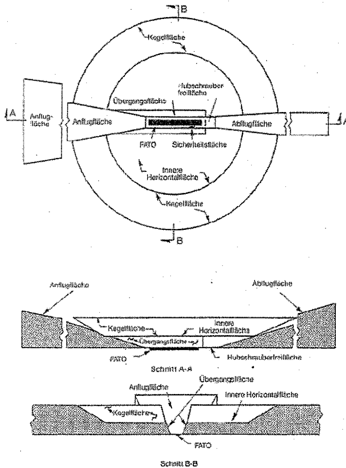
Abb. 4-1. Hindernisbegrenzungsflächen
